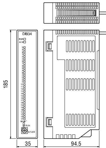
■ TC-net I/O module (Unit:mm)
