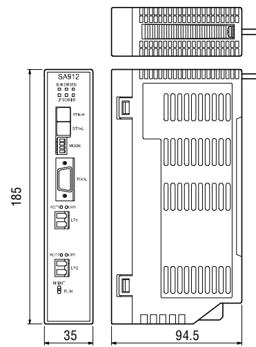
■ TC-net I/O adapter (Unit:mm)
